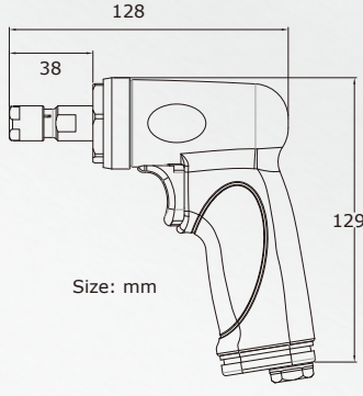
71106 Pistol Type 1/4" Die Grinder
